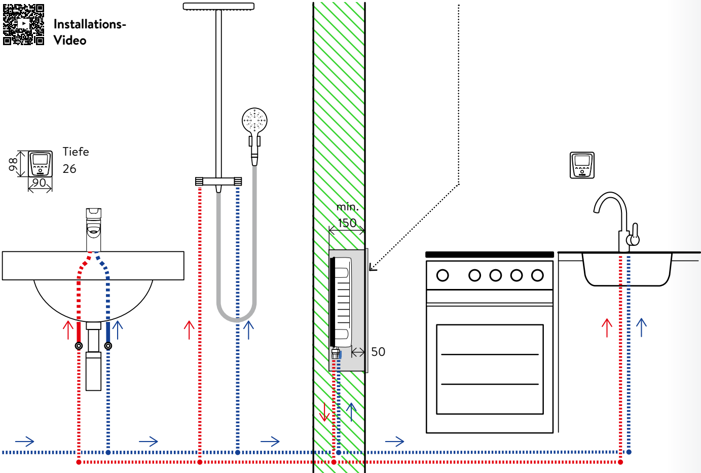
Maßangaben in mm | Installationsbeispiel einer Unterputzinstallation in einer Vollwand mit Standard-Revisionsklappe (bei Trockenbauwänden Abweichungen möglich – siehe Montageanleitung).
